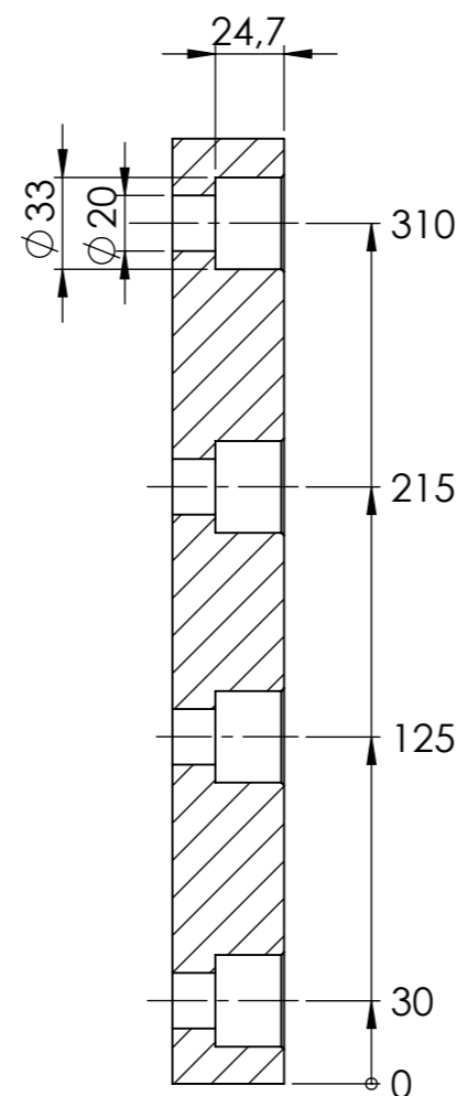
PRZEKRÓJ A-A SKALA 1 : 3
