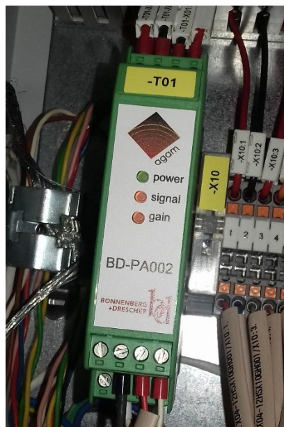
Preamplifier (przedwzmacniacz) BD-PA002
